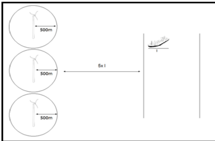
Rys. 9 Określenie odległości bezpiecznej pomiędzy zewnętrzną granicą toru wodnego/TSS a farmą wiatrową
