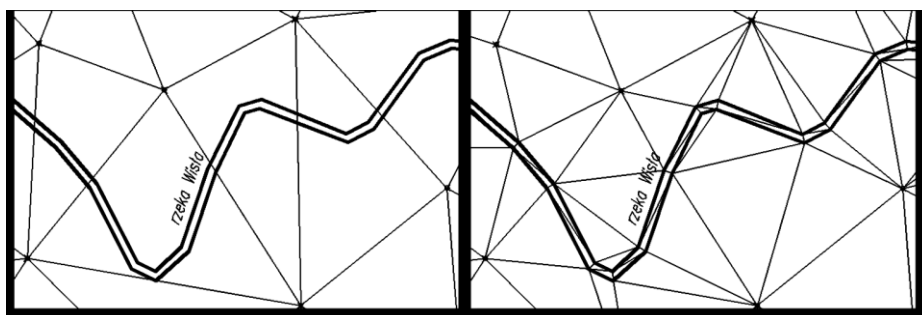
Rys. 1 Efekt wprowadzenia linii nieciągłości do modelu
