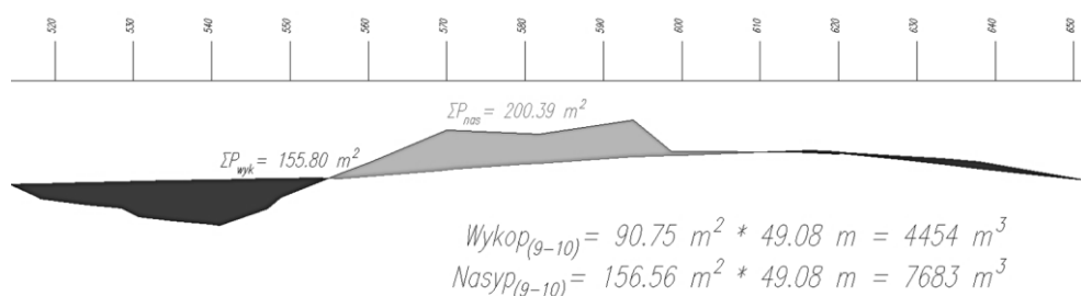
Rys. 12 Wykres z zaznaczonymi: wykopem i nasypem utworzonym poleceniem WykSPP
