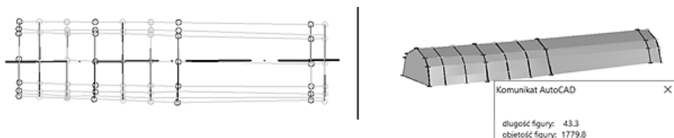
Rys. 9 Model przestrzenny wyrobiska
