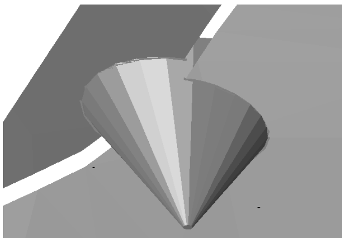
Rys. 7 Przecięcie się powierzchni filara spągu i szybu
