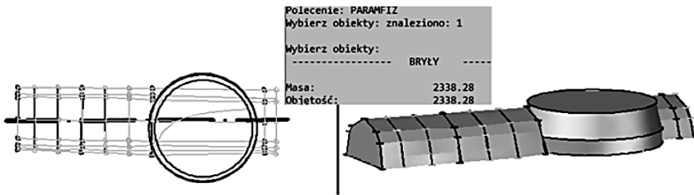
Rys. 10 Bryła obrazująca podszybie i szyb
