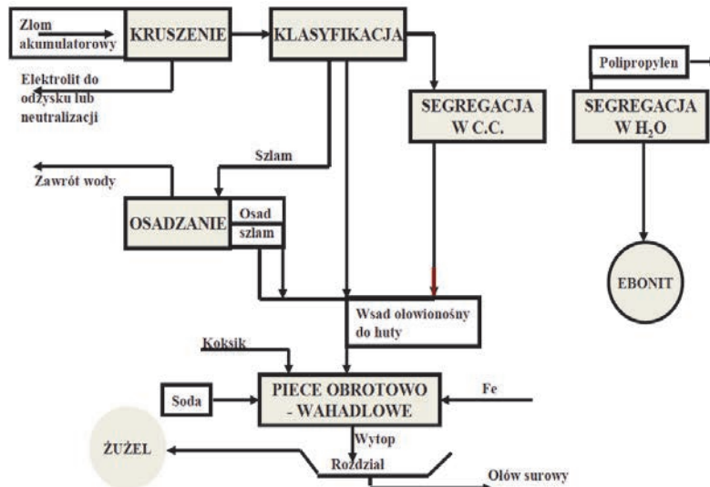
Rys. 4. Przykładowy schemat technologiczny przerobu złomu akumulatorowego Fig. 4. Example of schema of battery scrap processing technology
